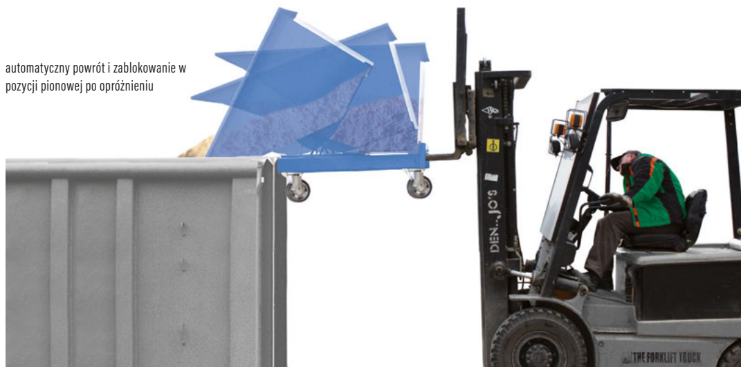
Koła poliuretanowe 92° Shore A nośność 1500 kg
